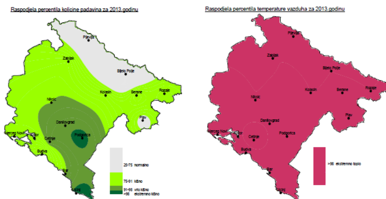
Slika 22. Raspodjelapadavina u Crnoj Gori u 2013.godini
