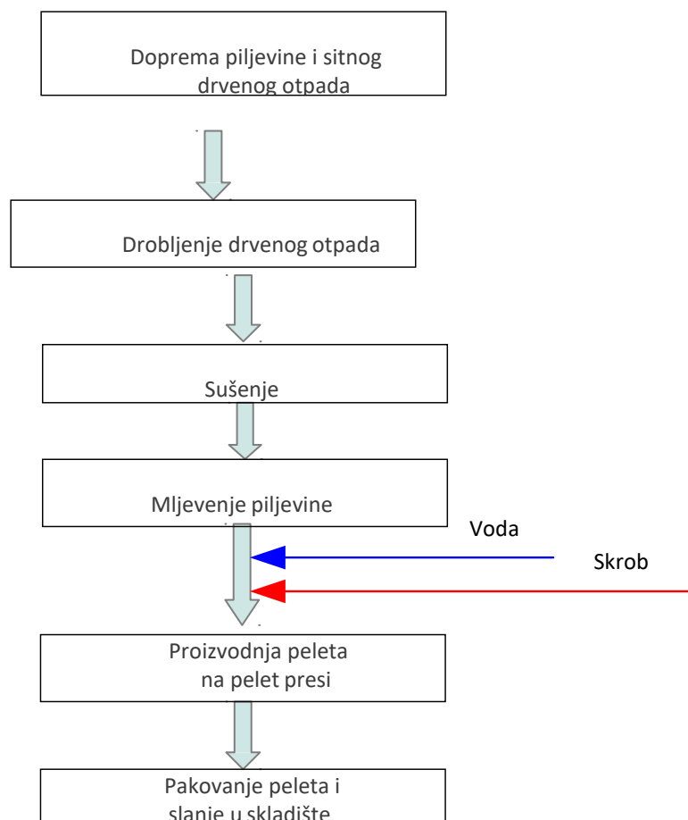
Sl.29. Diagram toka proizvodnje peleta:
