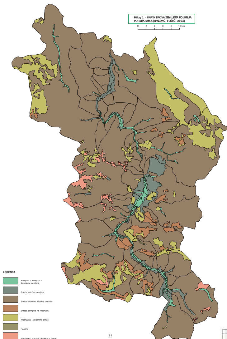
Slika 26. Pedološka karata Sliva rijeke Lim, Spalević i Fuštić, 2003.
