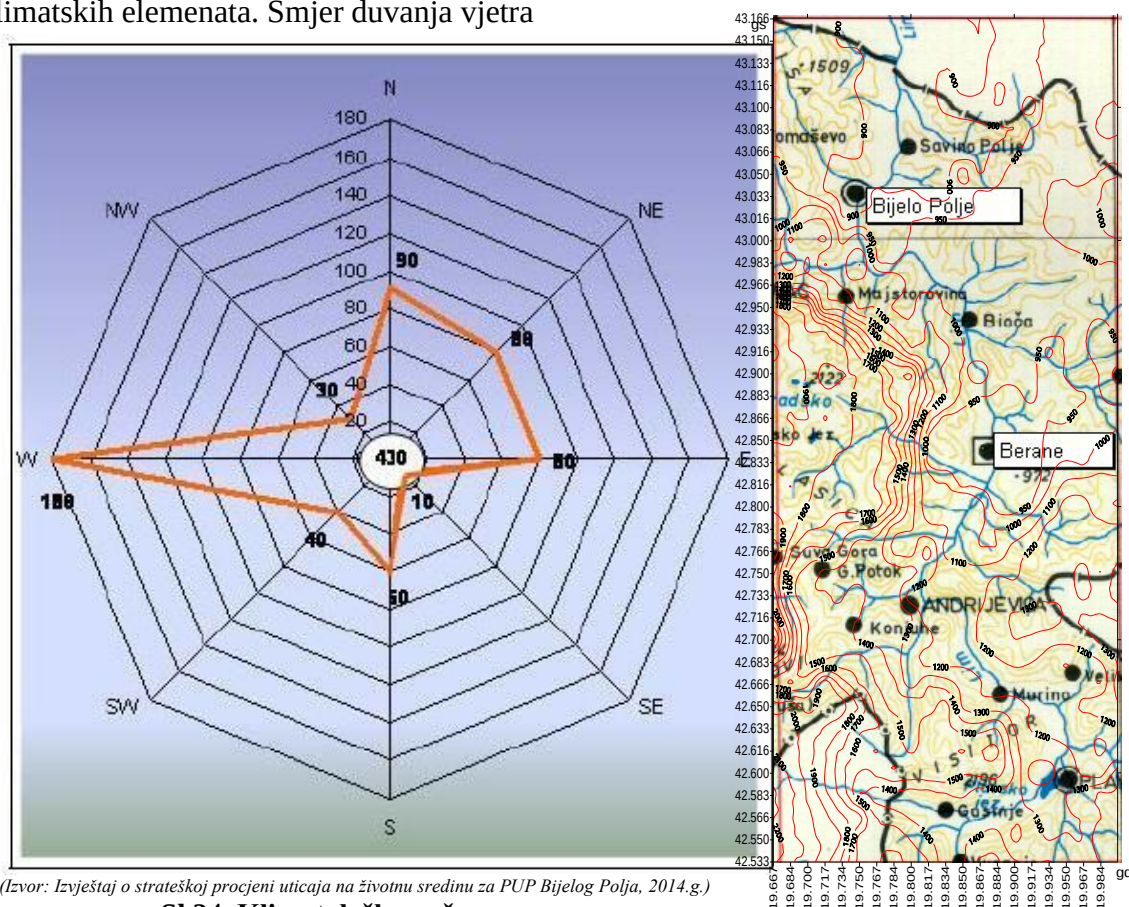
Sl.24. Klimatološka ruža
