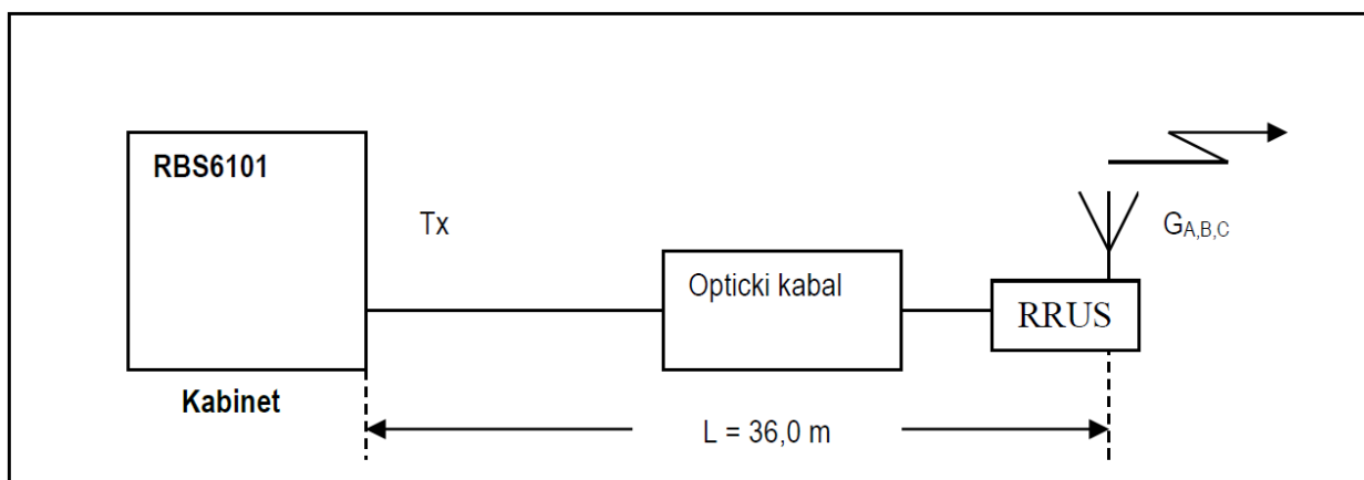
Skica: Proračun efektivne izračene snage
